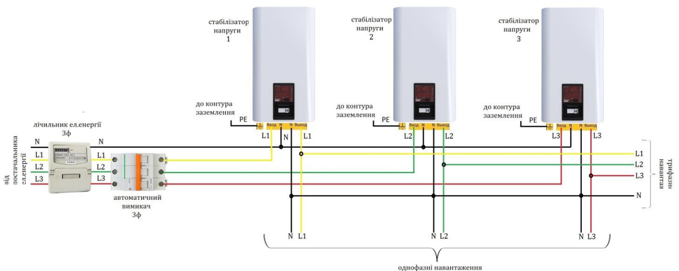
Рисунок 8. Схема підключення стабілізатора до трифазної мережі
